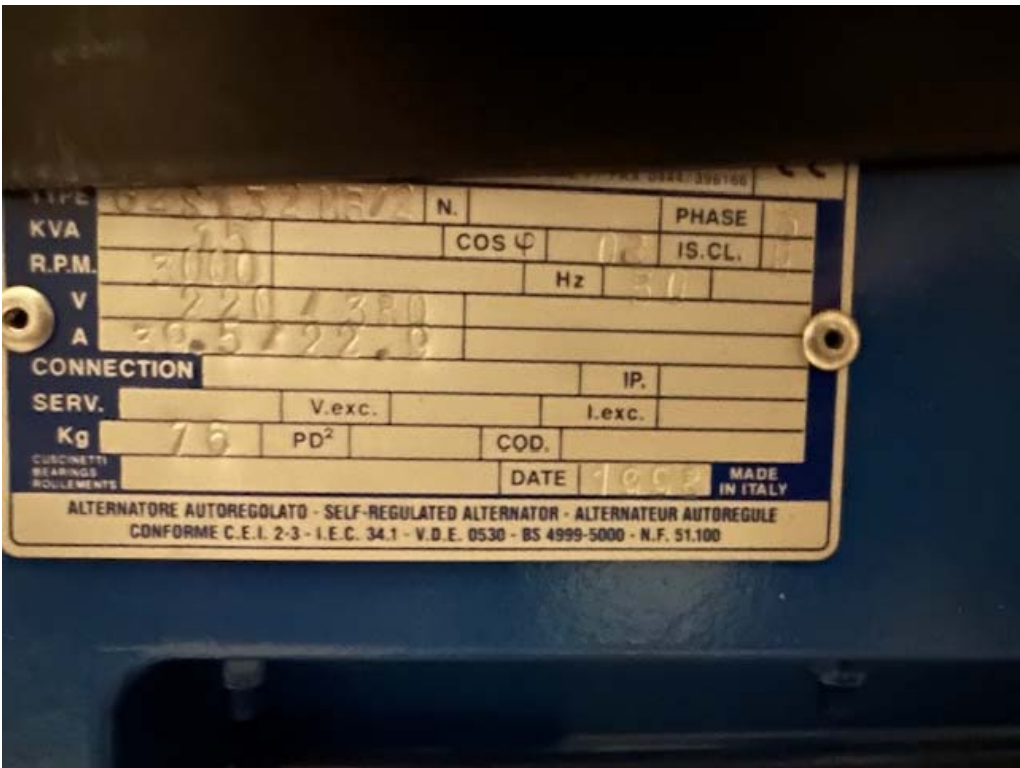
Allegato A3 – Targhetta identificativa gruppo elettrogeno
